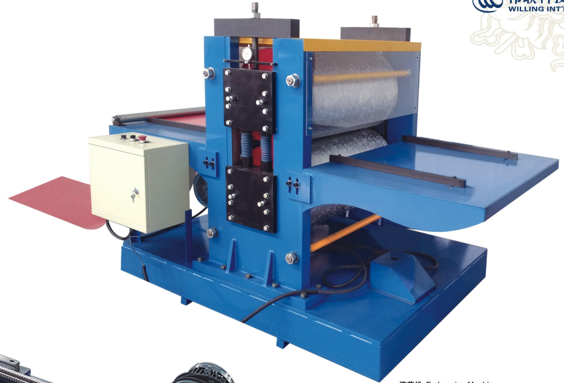
滚花机 Embossing Machine
